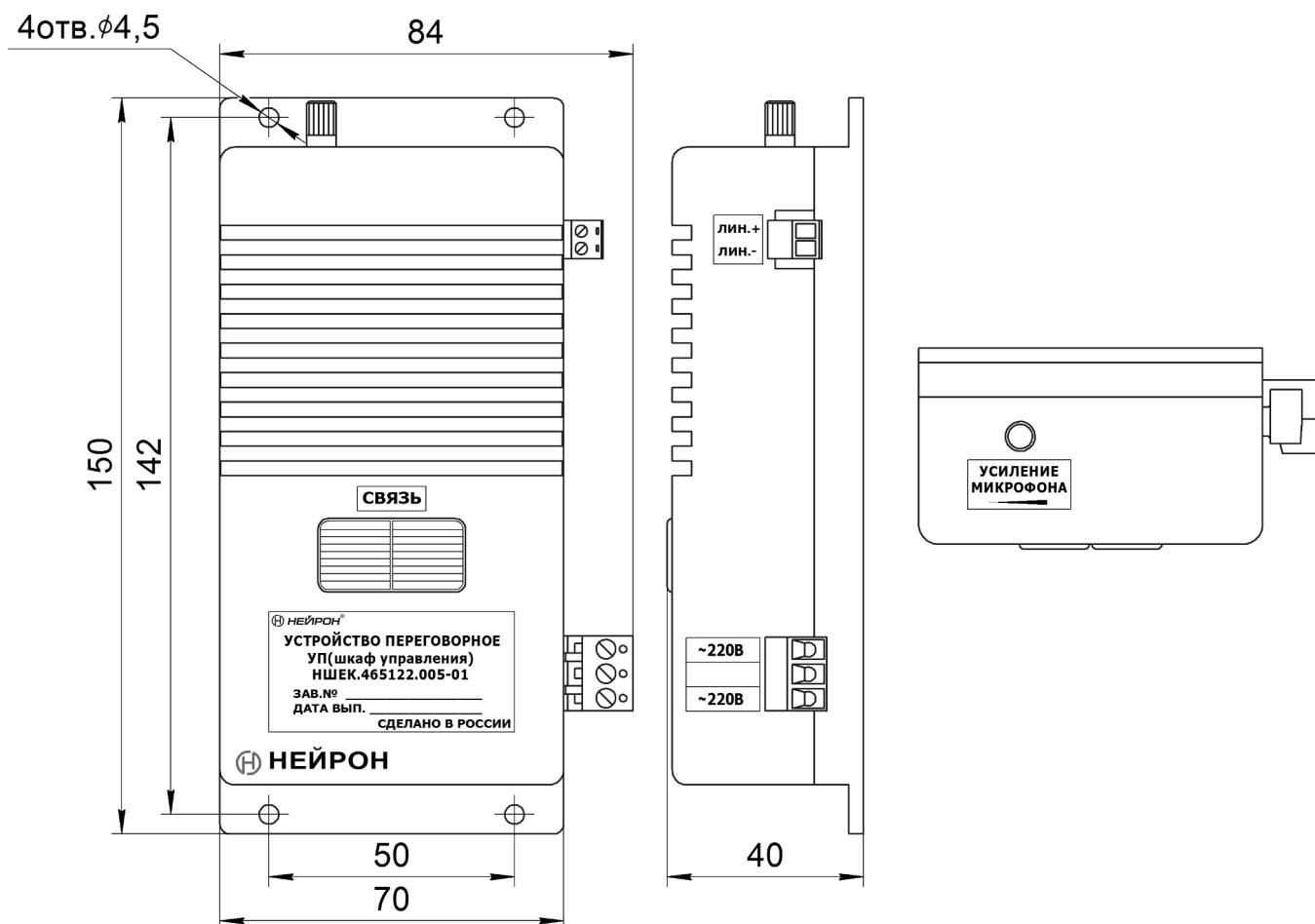
Рис.1 Внешний вид Устройство переговорное «УП(шкаф управления)» НШЕК.465122.005-01
